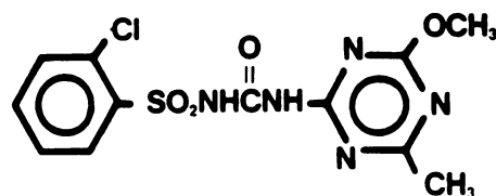
Chlorsulfuron
