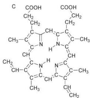
Protoporphyrin
