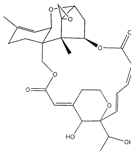
FIG. 9. Satratoxin H.
