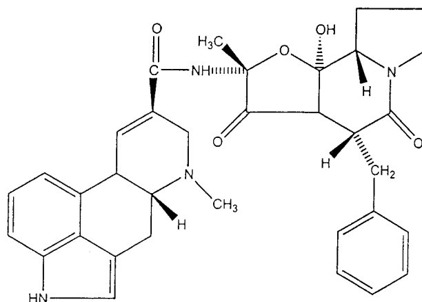
FIG. 3. Ergotamine.
