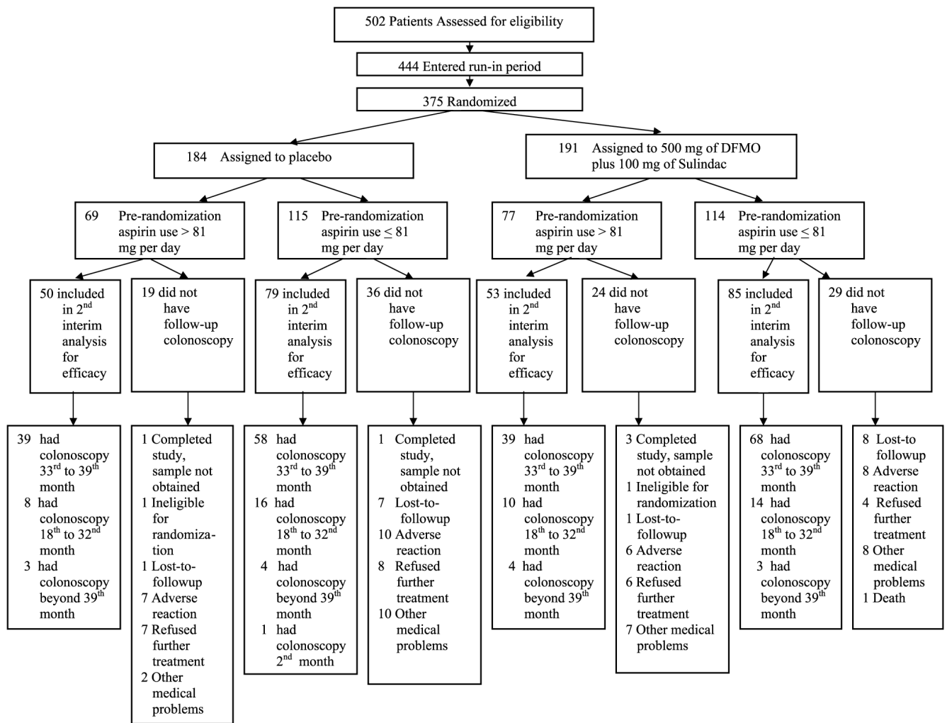
Fig. 1. Study schema.
