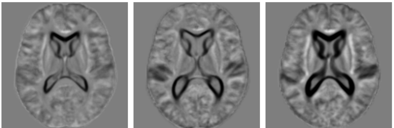
(d) Template 1 minus Template 2 (e) Template 2 minus Template 3 (f) Template 1 minus Template 3
