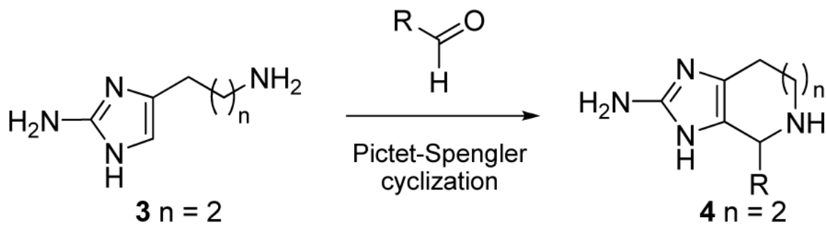
Scheme 1. Pictet-Spengler cyclization of 2-aminoimidazoles
