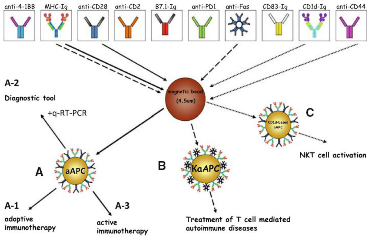
Fig. 1. The aAPC-“Lego-like”-system
