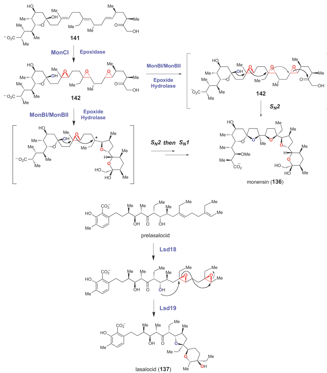
Scheme 21.
