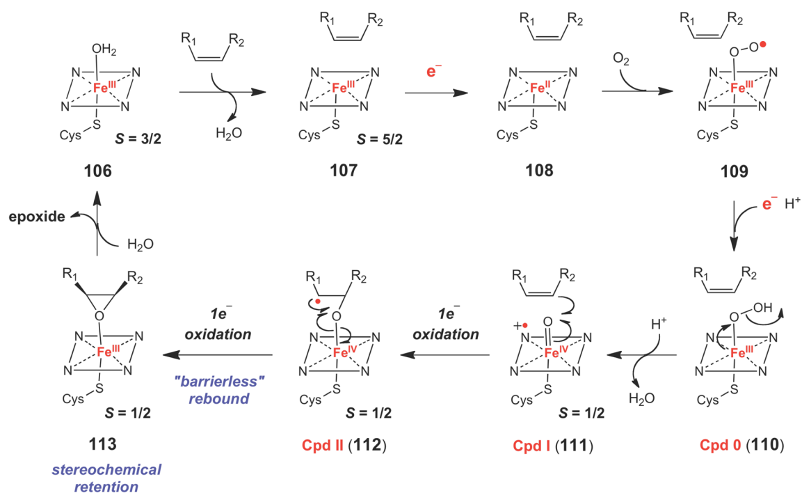
Scheme 16.
