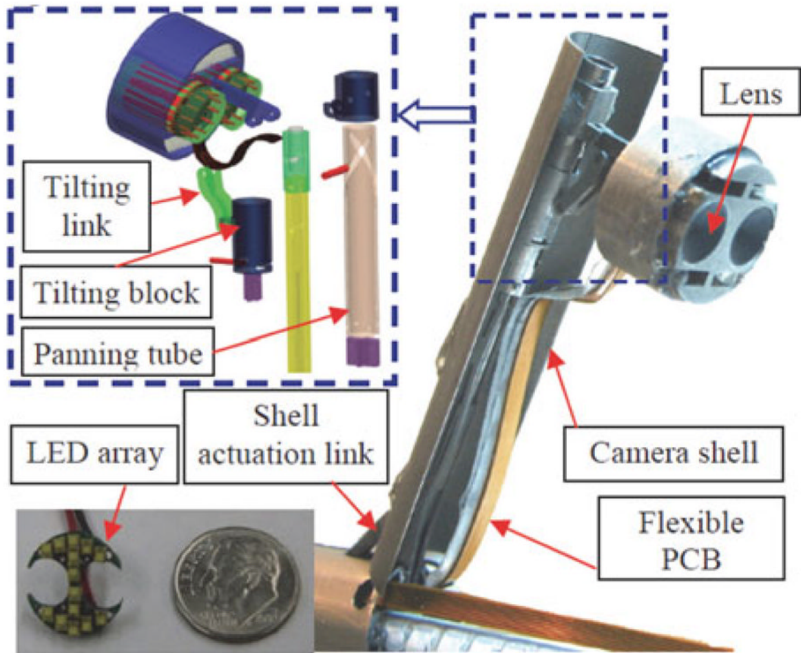
Fig. 16. Camera module of the IREP.
