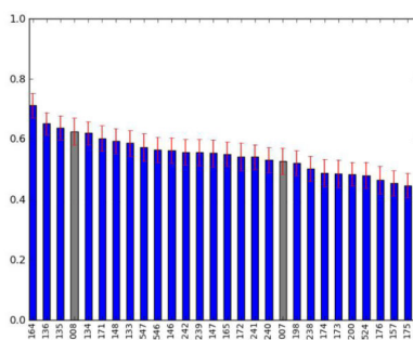
(b) AUC
