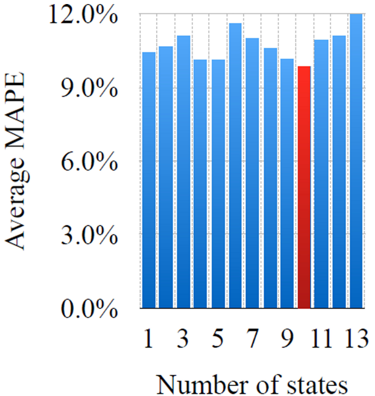
Figure 3. LDS EM overfitting in benchmark data.
