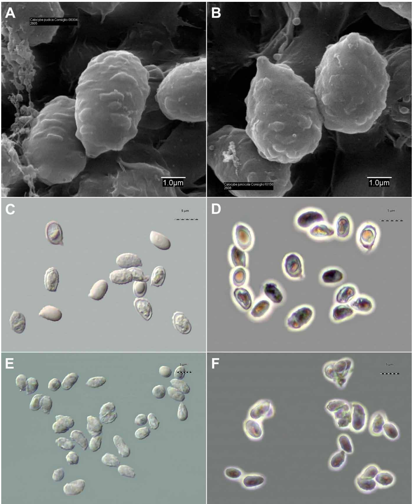
Fig. 4. Calocybella pudica . Spores. A, C–D (AMB 15995). B (AMB 15997). E–F (LIP-MB 991027 – isotype). Bars: A–B = 1 \mu\text{m} , C–F = 5 \mu\text{m} .
