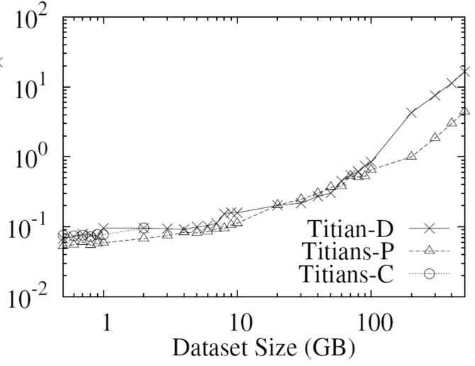
(d) WordCount Titian versions
