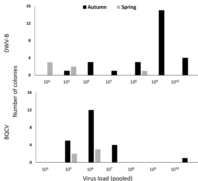
Figure 2. Histogram of DWV-B and BQCV viral titre in pooled colony samples (N = 30 bees per colony). Values represent average titre per bee. Black: viral titres in autumn; grey: viral titres in spring.
