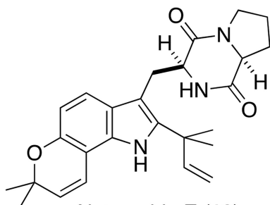
Notoamide E (12)
