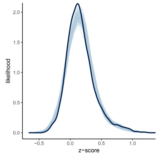
(b) BML posterior predictive density
