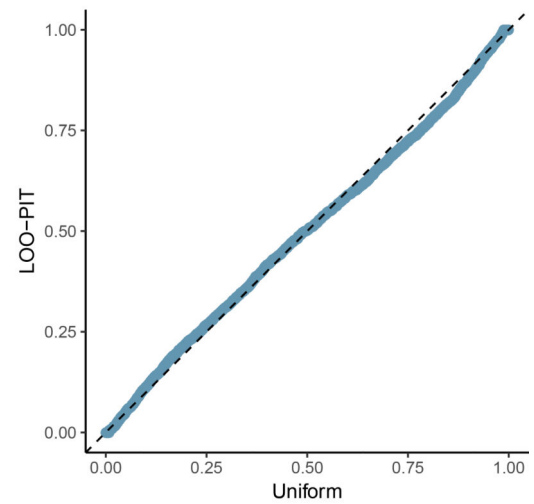
(d) BML cross-validation: Q-Q plot (uniform)
