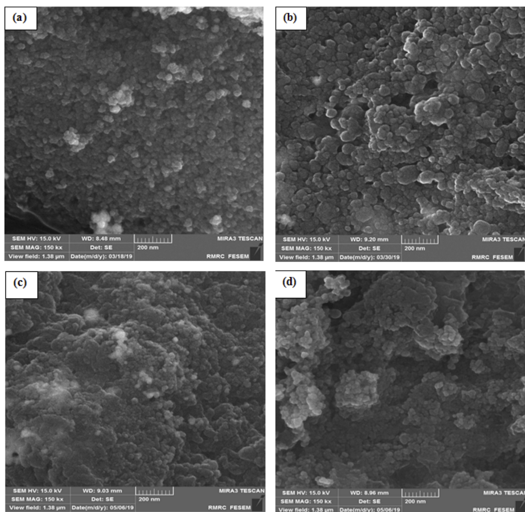
Figure 7 FE-SEM result of (A) \gamma -Fe 2 O 3 @Au/PβCD, (B) \gamma -Fe 2 O 3 @Au/PβCD/PAA-SDN, (C) \gamma -Fe 2 O 3 @Au/PβCD/PAA-SDN/PEI-βCD and (D) nanocapsule.
