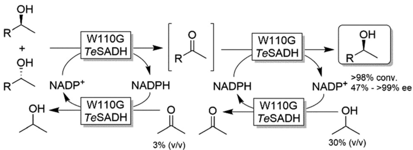
Scheme 17.
