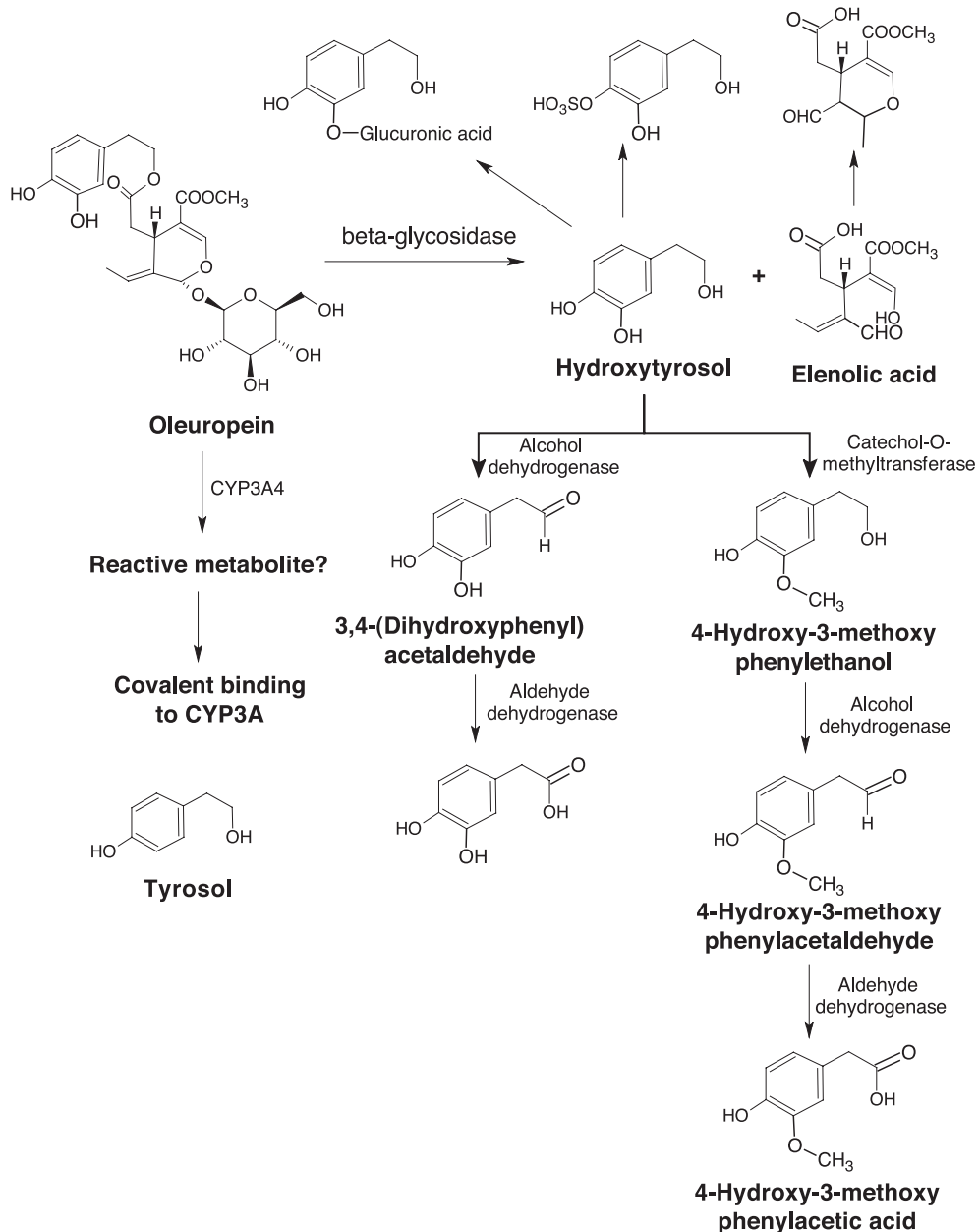
Fig. 10. Metabolism of oleuropein.
