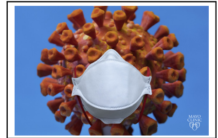
SARS-CoV-2.
