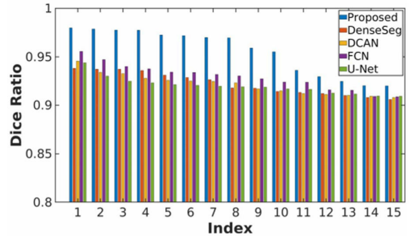
(f) Rectum: The worst 15.
