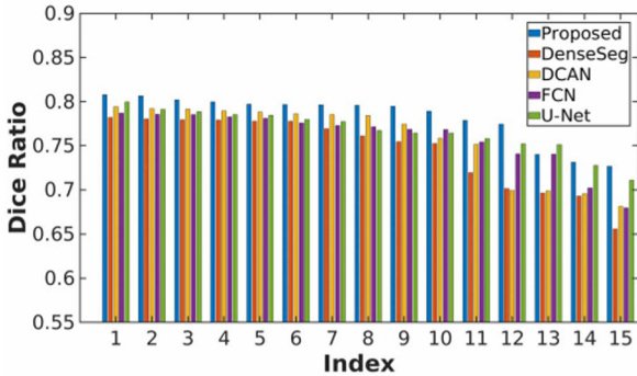
(e) Rectum: The top 15.
