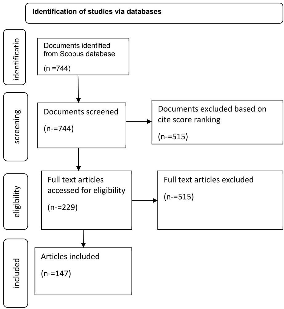
Fig. 1. PRISMA diagram.
