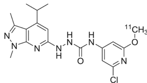
[ 11 C]TZ34125
