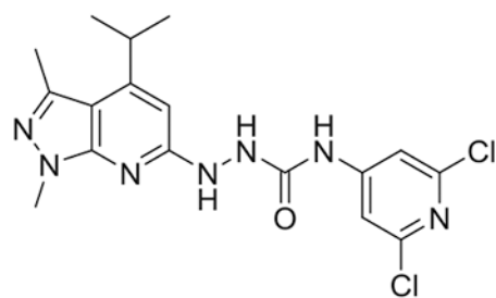
JTE-013
