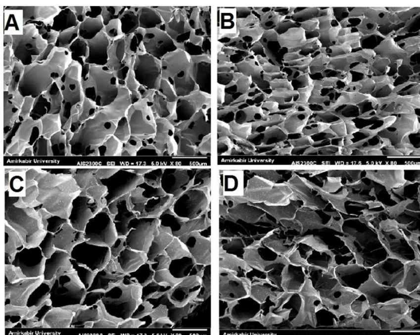
Fig. 2. SEM micrograph of (A) ALG, (B) ALG/RIS, (C) ALG/PLGA and (D) ALG/PLGA/RIS.
