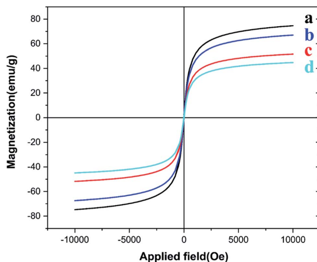
Fig. 9 VSM analysis of (a) \text{Fe}_3\text{O}_4 , (b) \text{Fe}_3\text{O}_4@CPTMS , (c) \text{Fe}_3\text{O}_4@PTMS\text{-}2,6\text{-diacetylpyridine} and (d) [\text{Fe}_3\text{O}_4@PAM\text{-Schiff base-Mn}][\text{ClO}_4] MNPs.
