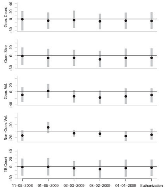
(f) IL7
