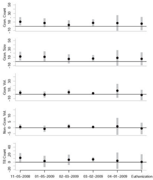
(g) IP10
