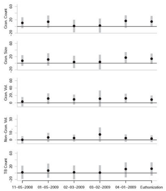
(h) NRAMP1
