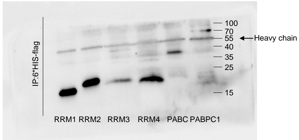
FigS5.B 15%GEL
