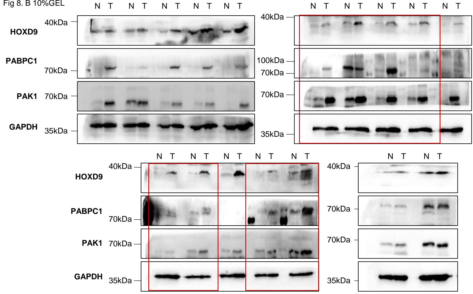
Fig 8. A 10%GEL
