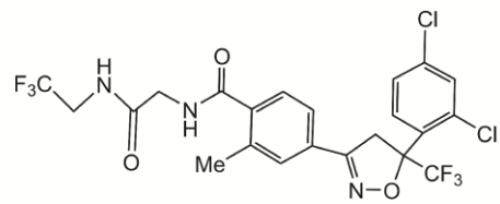
2010 Fluralaner isoxazoline
