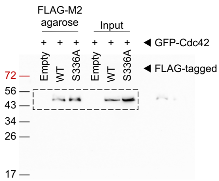
Fig 6b. FLAG
