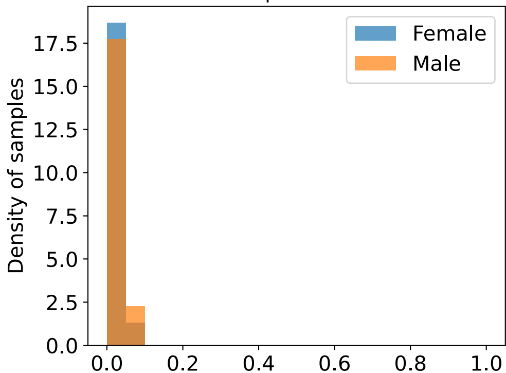
Epoch: 25
