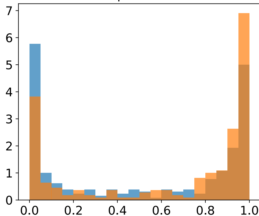
Epoch: 100
