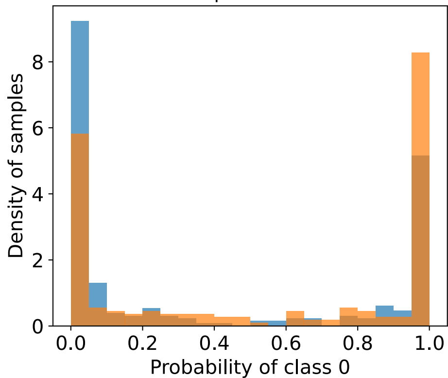
Epoch: 25
