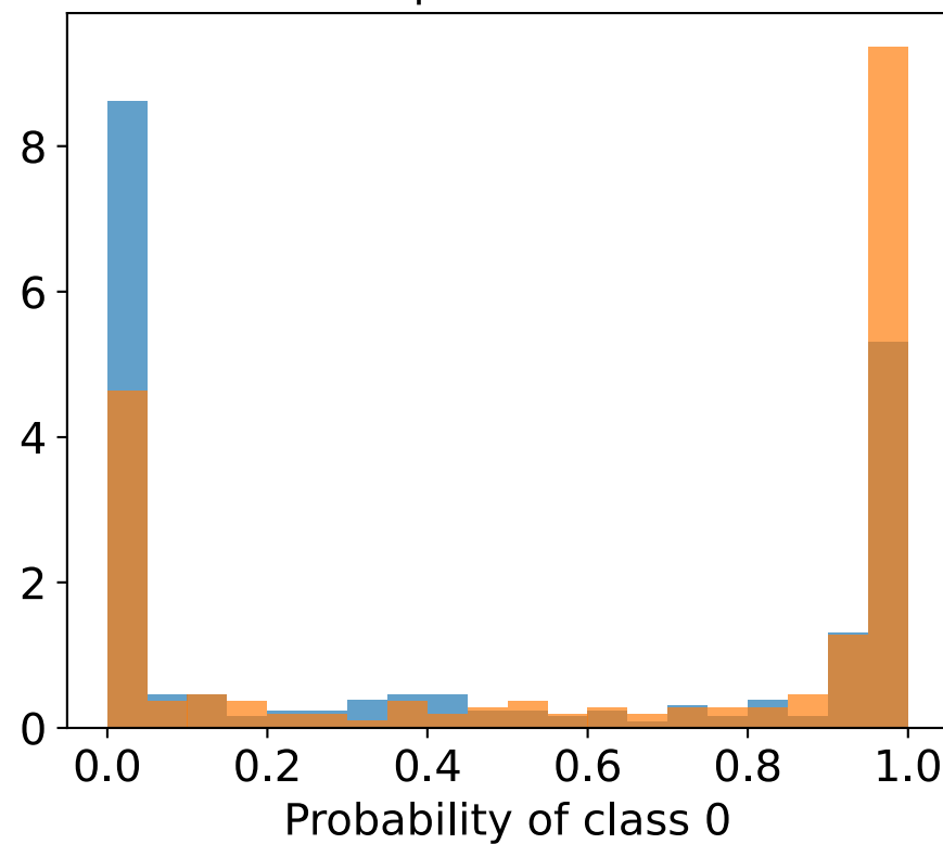
Epoch: 100
