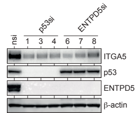
c H1975 (NSCLC) p53 R273H
