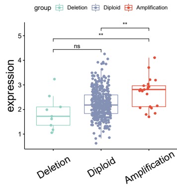
E TET2_ANOVA_tests:p=0.257
