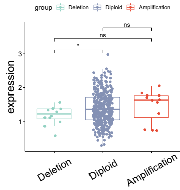
E TET2_ANOVA_tests:p=0.257
