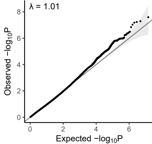
ChrX CN-LOH
