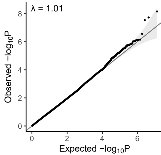
ChrX All
