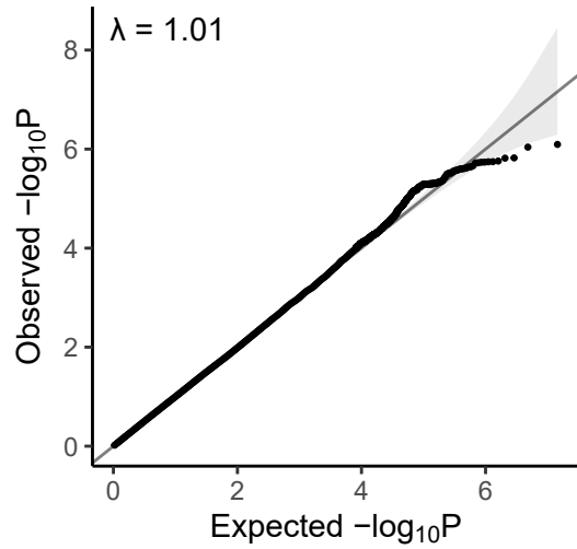
Autosomal CN-LOH
