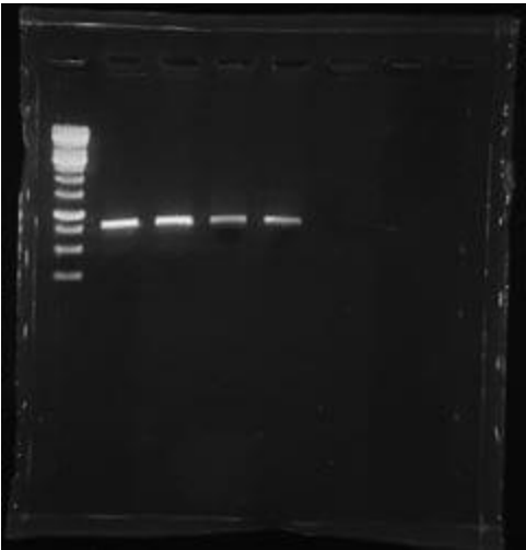
PESN1
