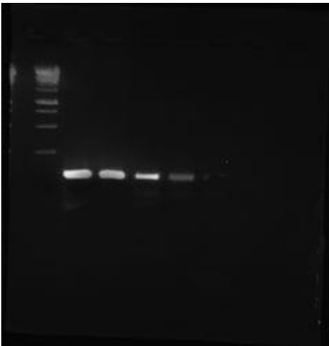
BACE1
