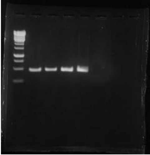
PESN1
