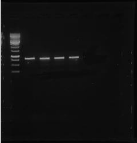
BACE1
