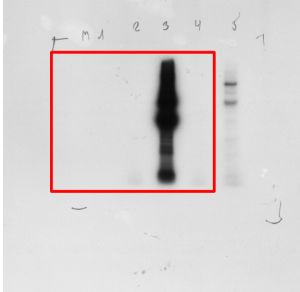
H9C2 autoradiogram
