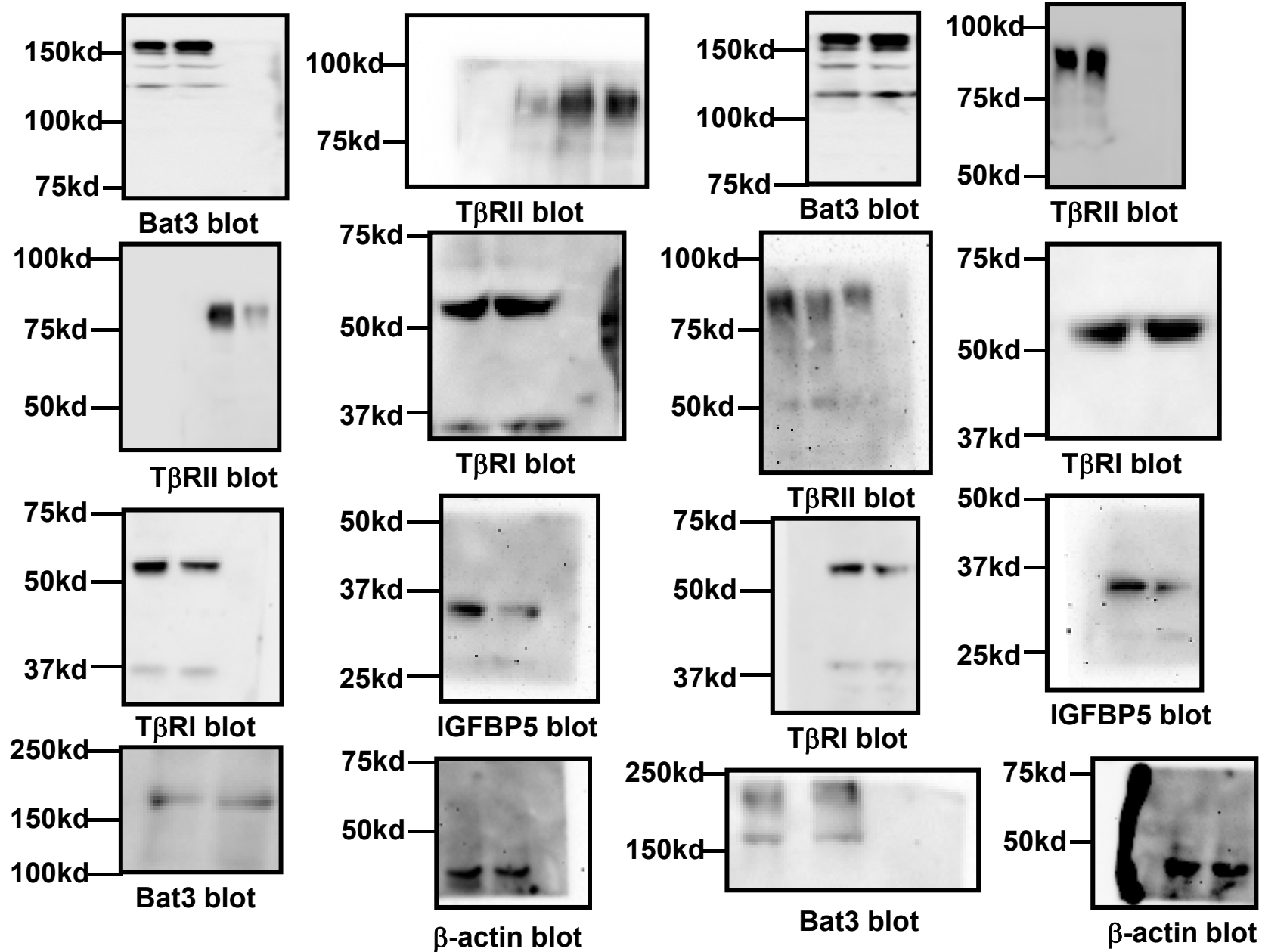
Figure 6G
