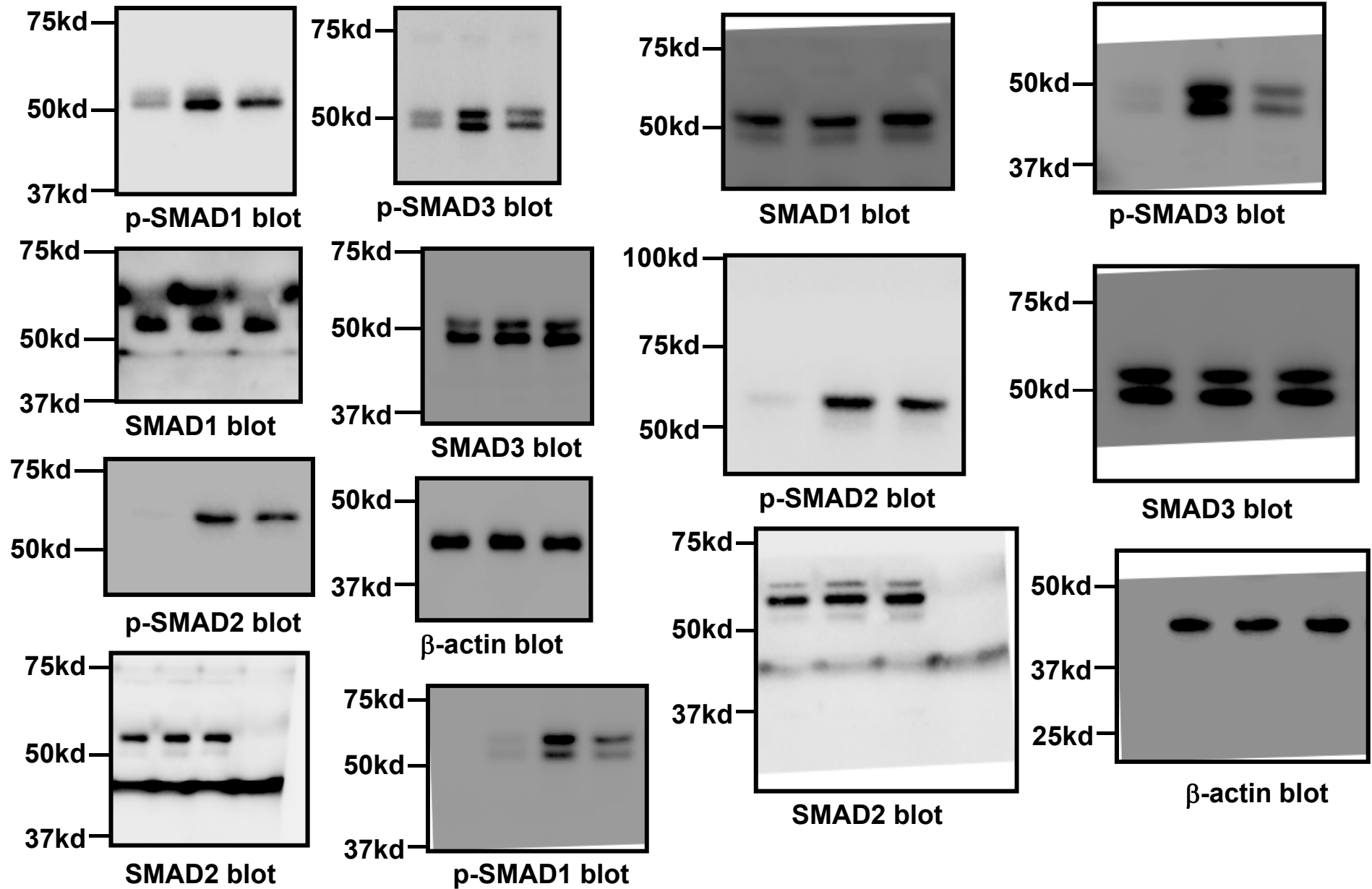
Figure 6E
