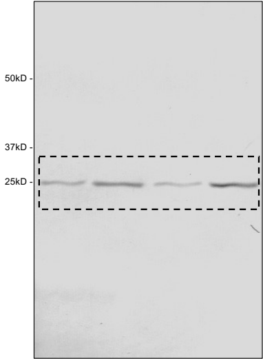
TFAM
