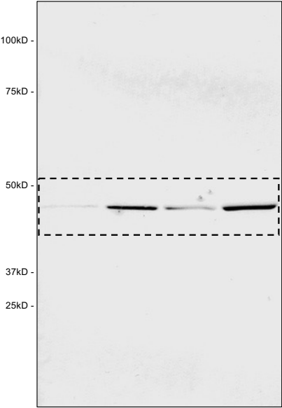
c-Jun
