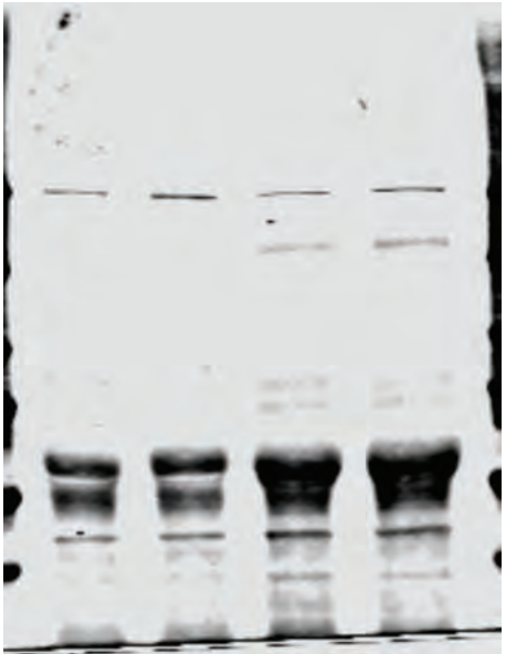
Propionylation
