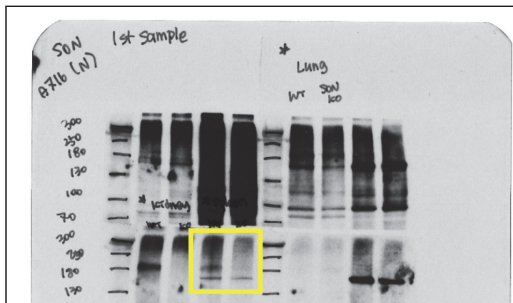
Spleen_Son
