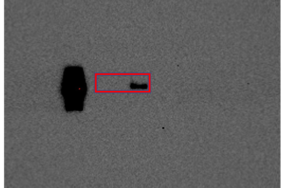
P62
