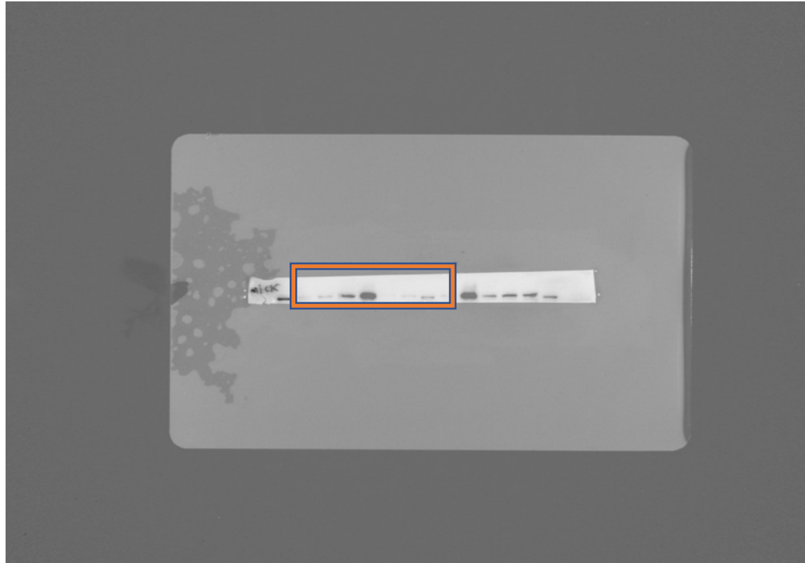
MLCK1
