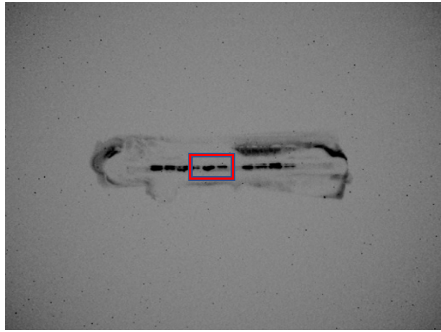
P62
