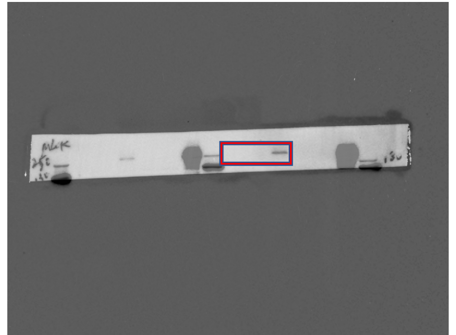
MLCK1
