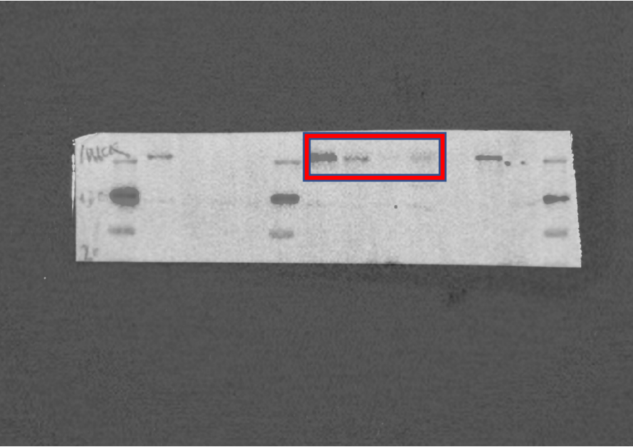
MLCK1
