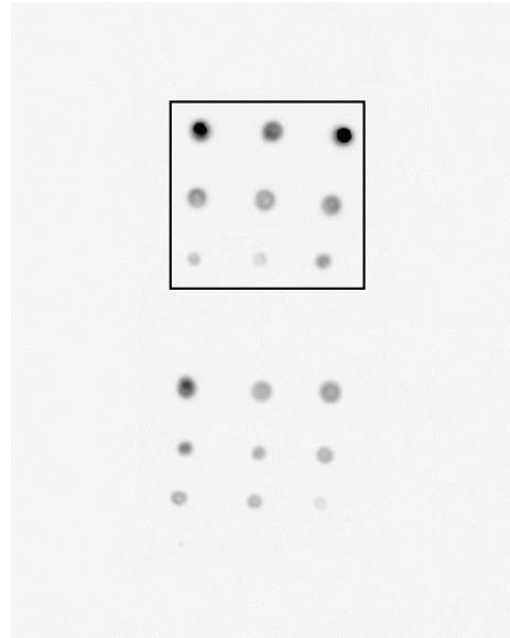
m6A
