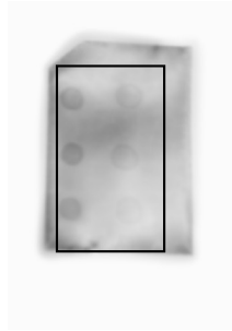
m6A
