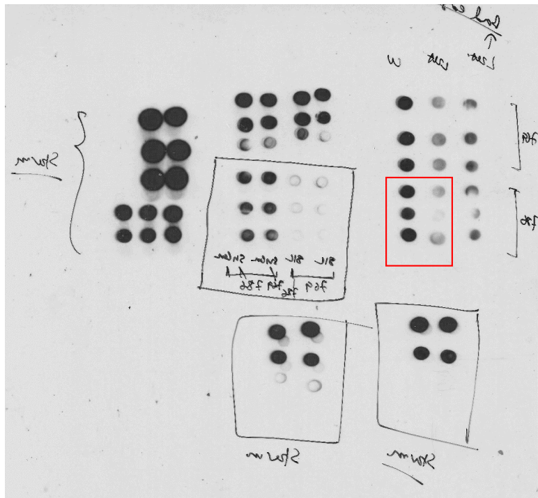
m6A
