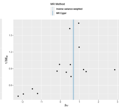
CD20-CD38-AC
