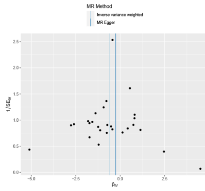
IgD-CD38-%lymphocyte
