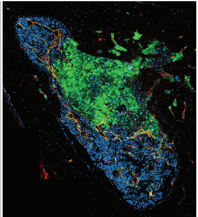
Lenvatinib
