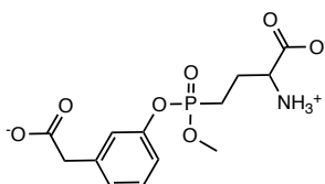
GGsTop (CAS: 926281-37-0)
