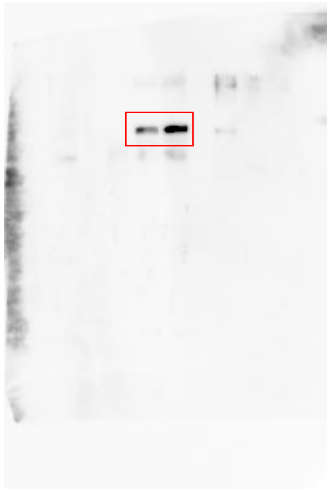
RhoA
