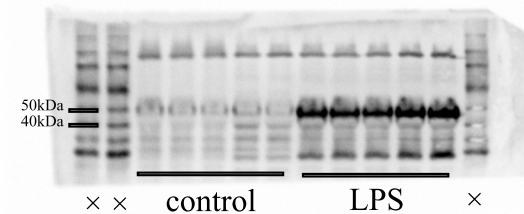
Orm1 47 kDa
