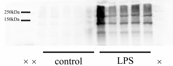
A2M 180 kDa
