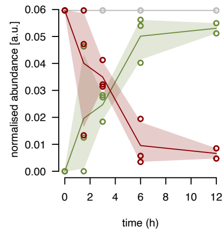
bL20m fraction 4
