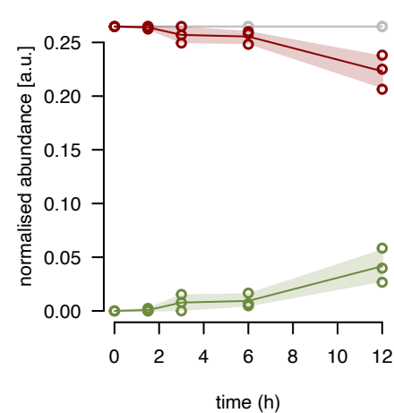
mL65 fraction 12
