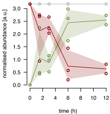
mL54 fraction 2
