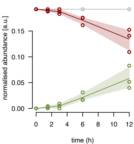
uL3m fraction 13
