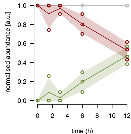
mL54 fraction 8
