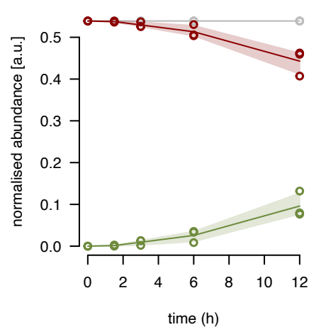
mL65 fraction 11
