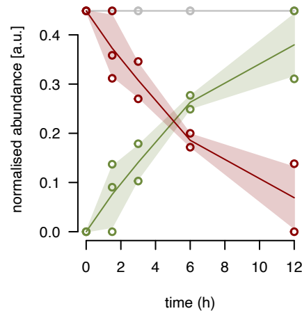
mL54 fraction 3
