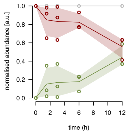
mL48 fraction 8
