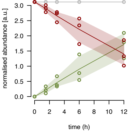
mL46 fraction 5
