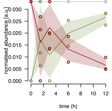
uL23m fraction 8
