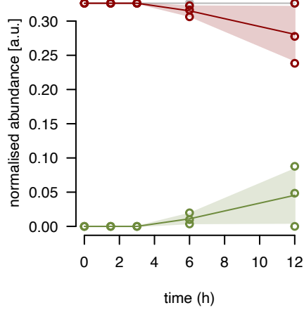
mL46 fraction 14
