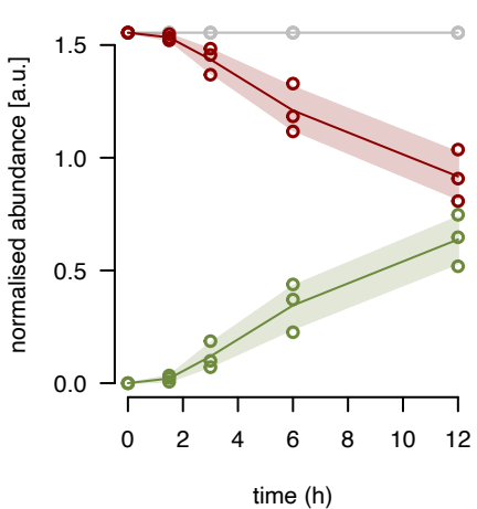
mL65 fraction 9
