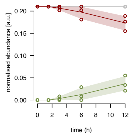
bL20m fraction 12
