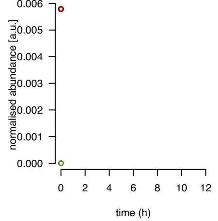
mL64 fraction 4
