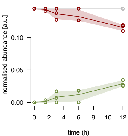
mL65 fraction 13
