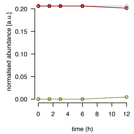
mL42 fraction 12
