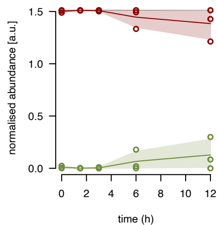
mL48 fraction 16
