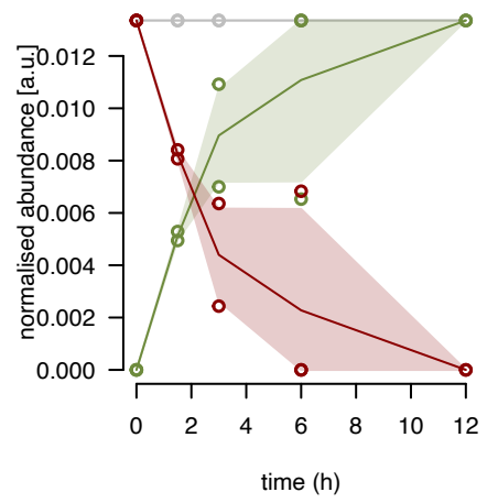
bL28m fraction 4
