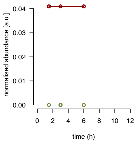
mL42 fraction 14
