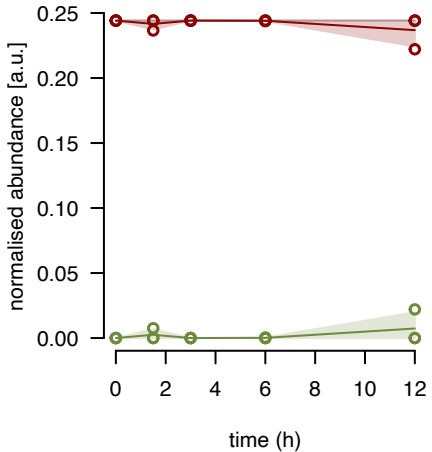
mL48 fraction 13
