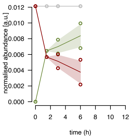
bL9m fraction 2
