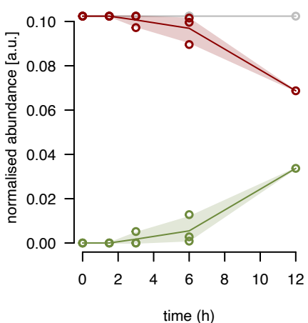
bL20m fraction 13
