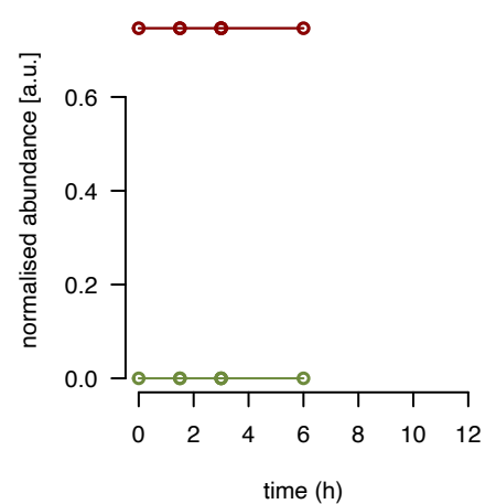
mL52 fraction 16
