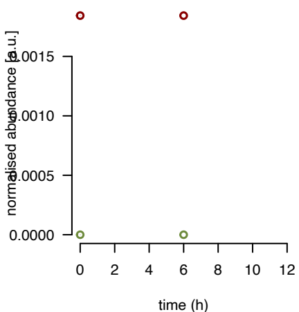
bL9m fraction 5
