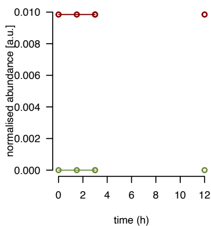
mL53 fraction 7
