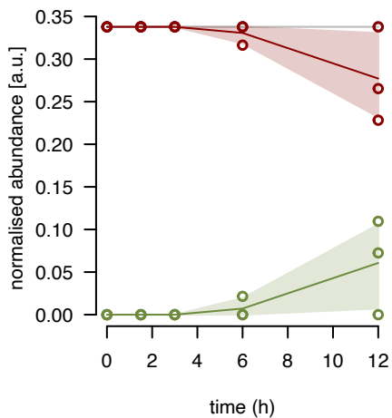
mL53 fraction 10
