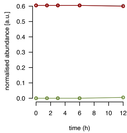
mL52 fraction 11
