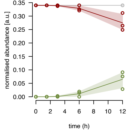
bL28m fraction 12
