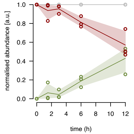
bL28m fraction 8
