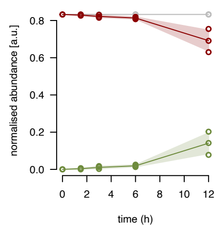
mL65 fraction 16
