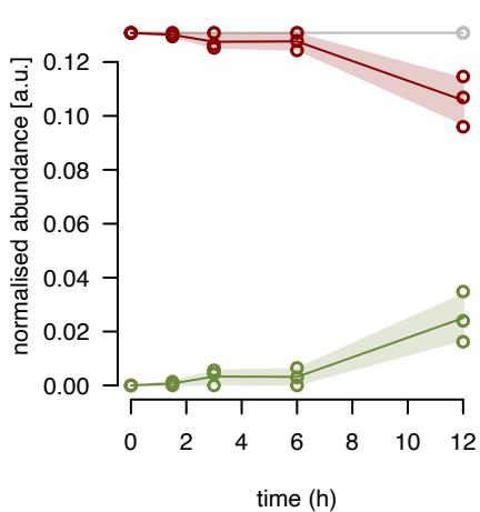
mL65 fraction 14
