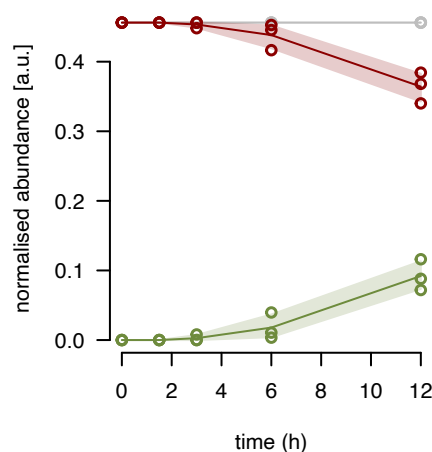
bL20m fraction 11
