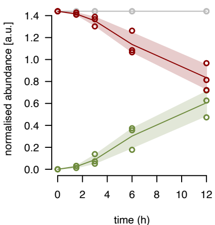
bL9m fraction 9
