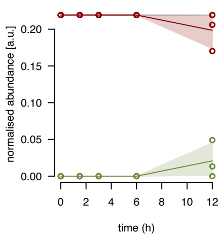
mL53 fraction 15
