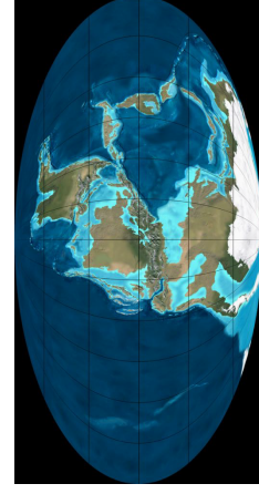
400 Mya
