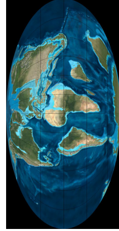
65 Mya
