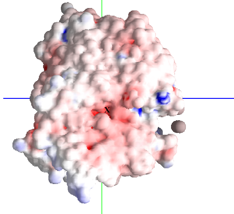
(b) AxNiR
