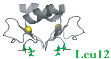
ZBD dimer
